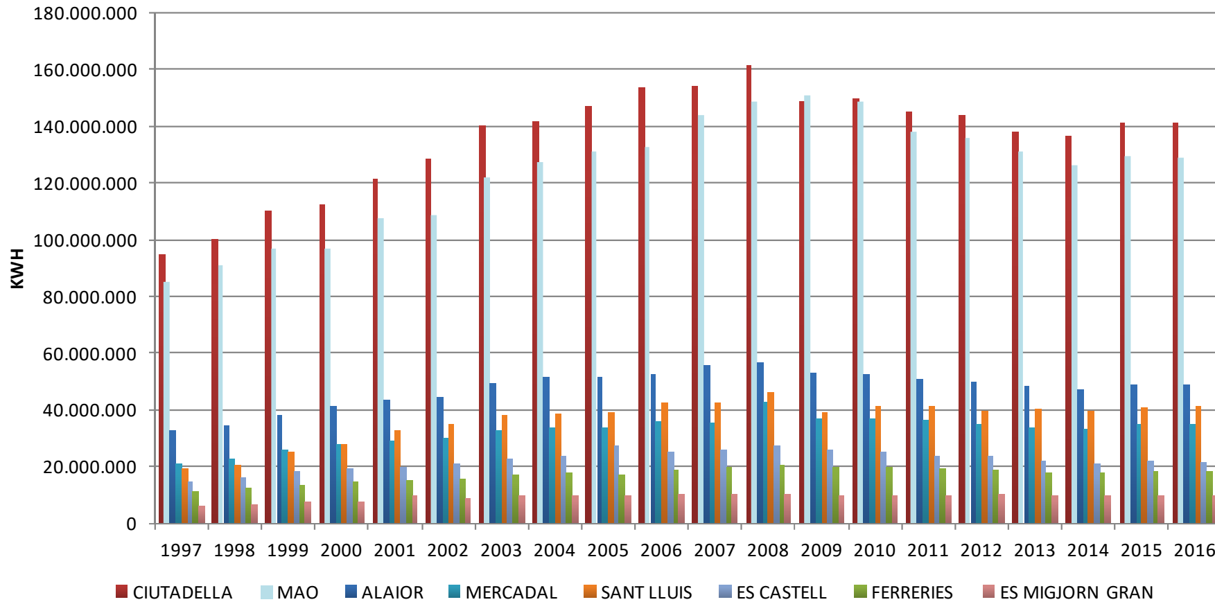
Gràfic 3. Evolució del consum elèctric anual per municipis. 1997-2016
