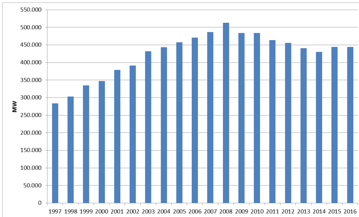
Gràfic 1. Evolució del consum elèctric anual al conjunt de l'illa. 1997-2016
